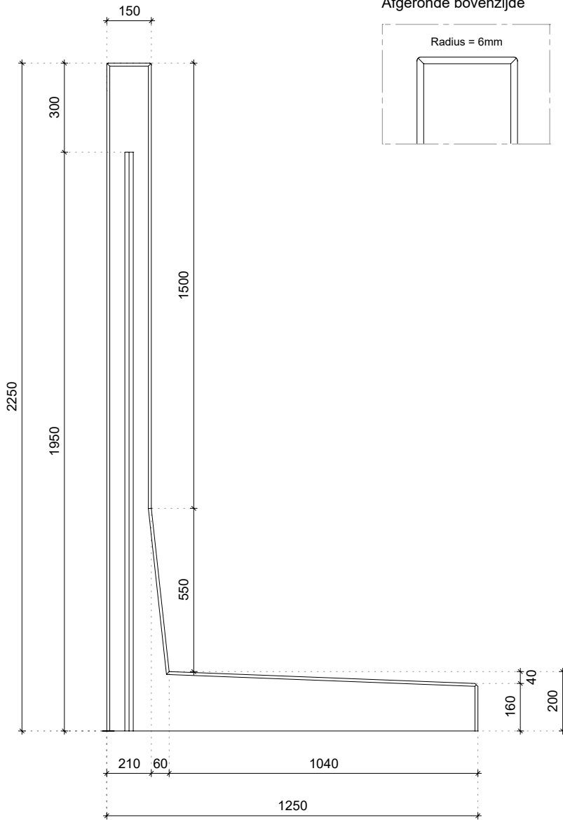
Afgeronde bovenzijde
