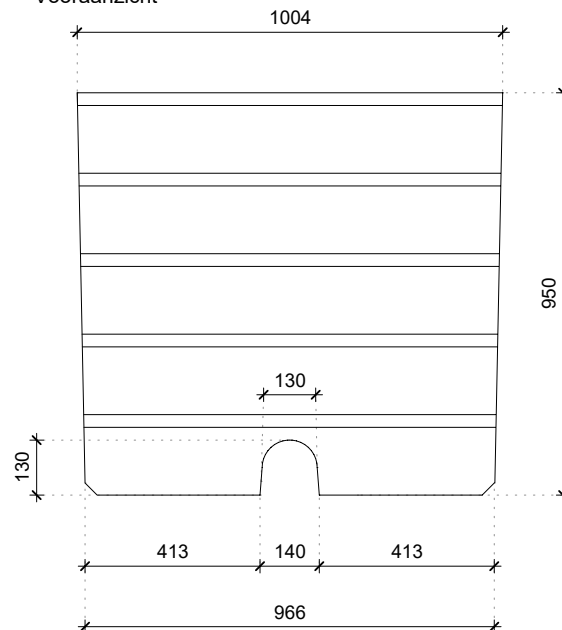
Vooraanzicht
