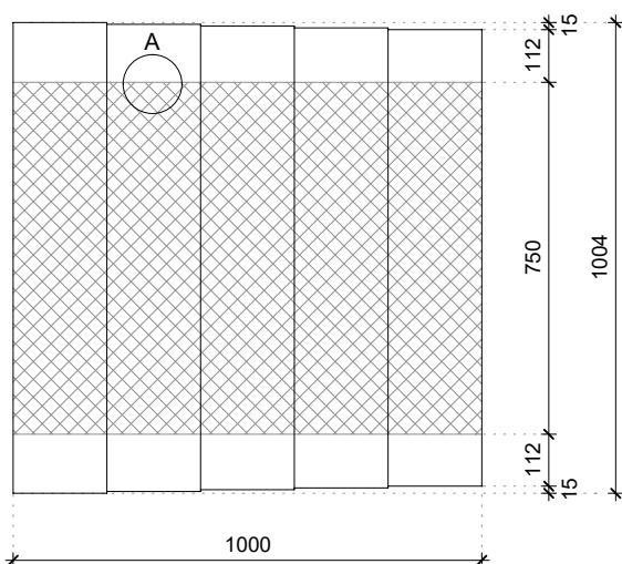
Bovenaanzicht
