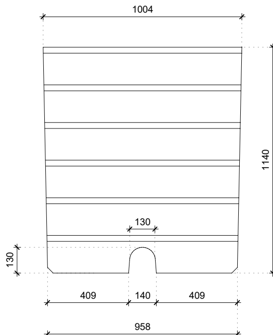
Vooraanzicht
