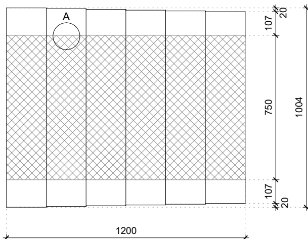
Bovenaanzicht
