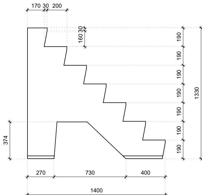
Zijaanzicht
