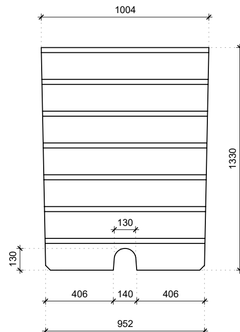
Vooraanzicht
